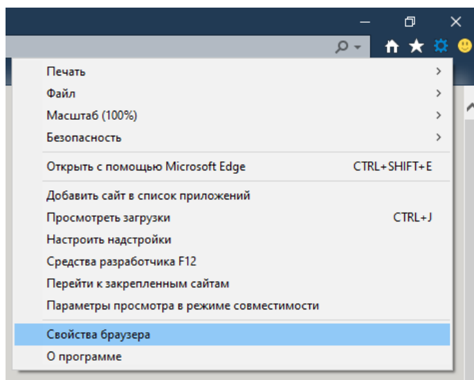
Рисунок 80 – Свойства браузера
