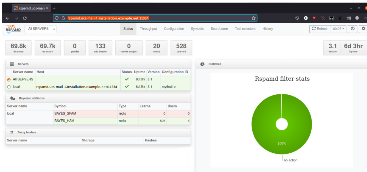
Рисунок 11 – Веб-интерфейс Rspamd
