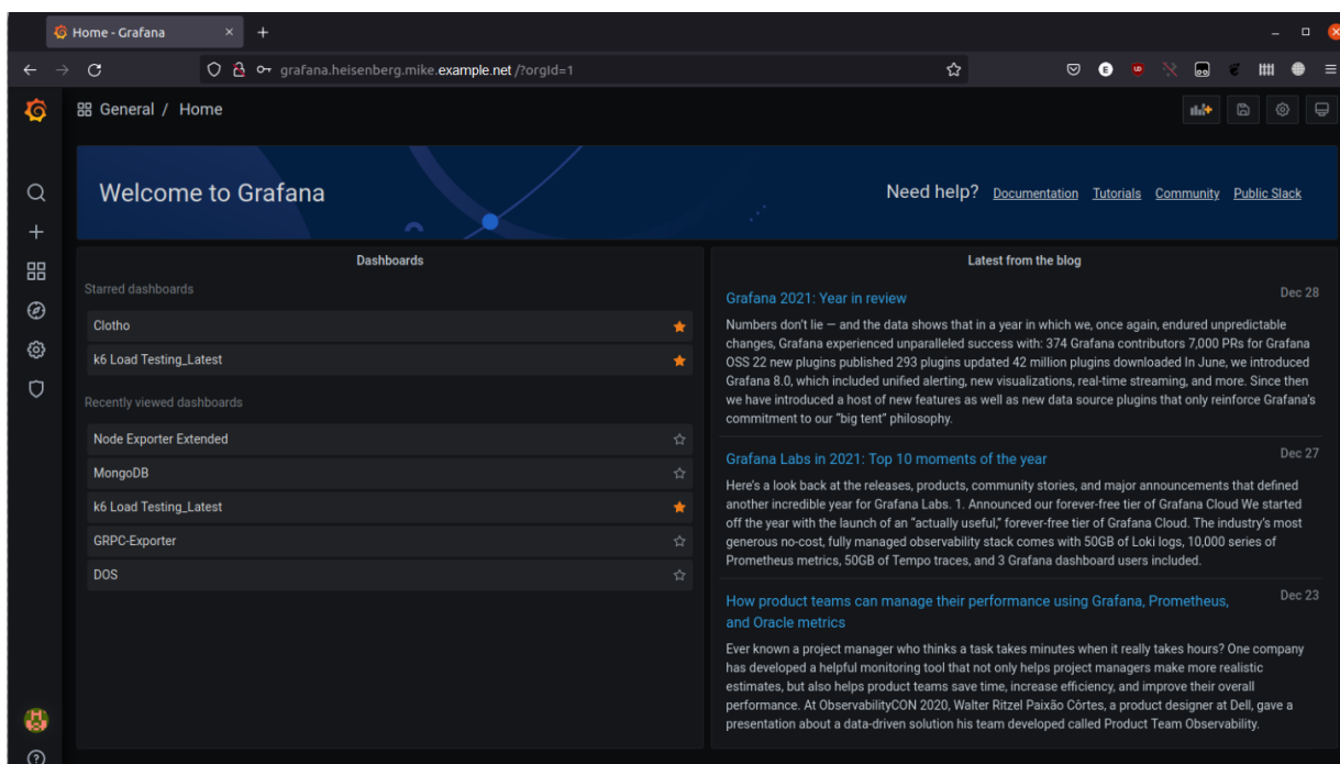
Рисунок 15 – Веб-интерфейс Grafana
