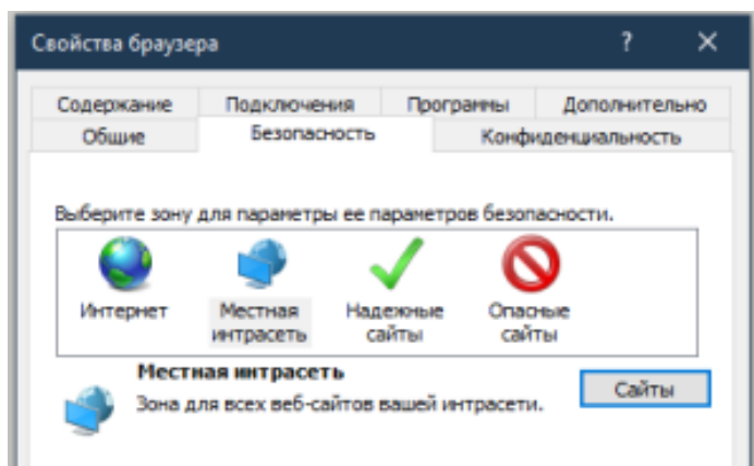
Рисунок 81 – Кнопка Сайты
